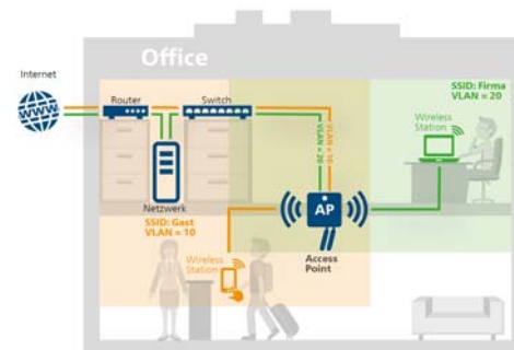
Fig. 4 : VLAN statique
