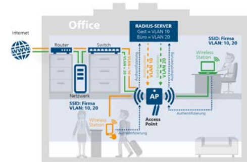
Fig. 5 : VLAN dynamique
